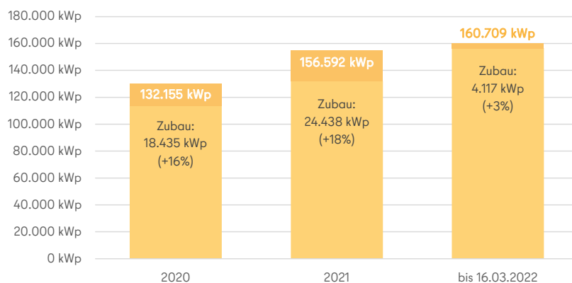
Abbildung 7 – Entwicklung der installierten PV-Leistung in Berlin
