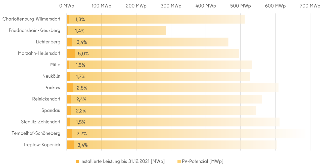
Abbildung 6 - Ausschöpfung des PV-Potenzials in den Berliner Bezirken
